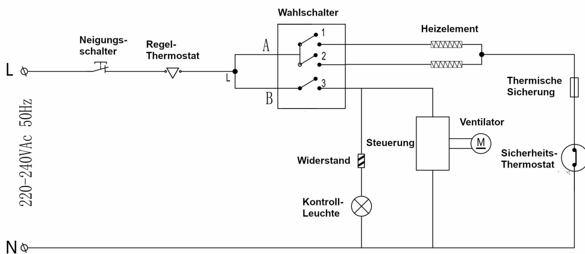
Schaltplan CH 2100
